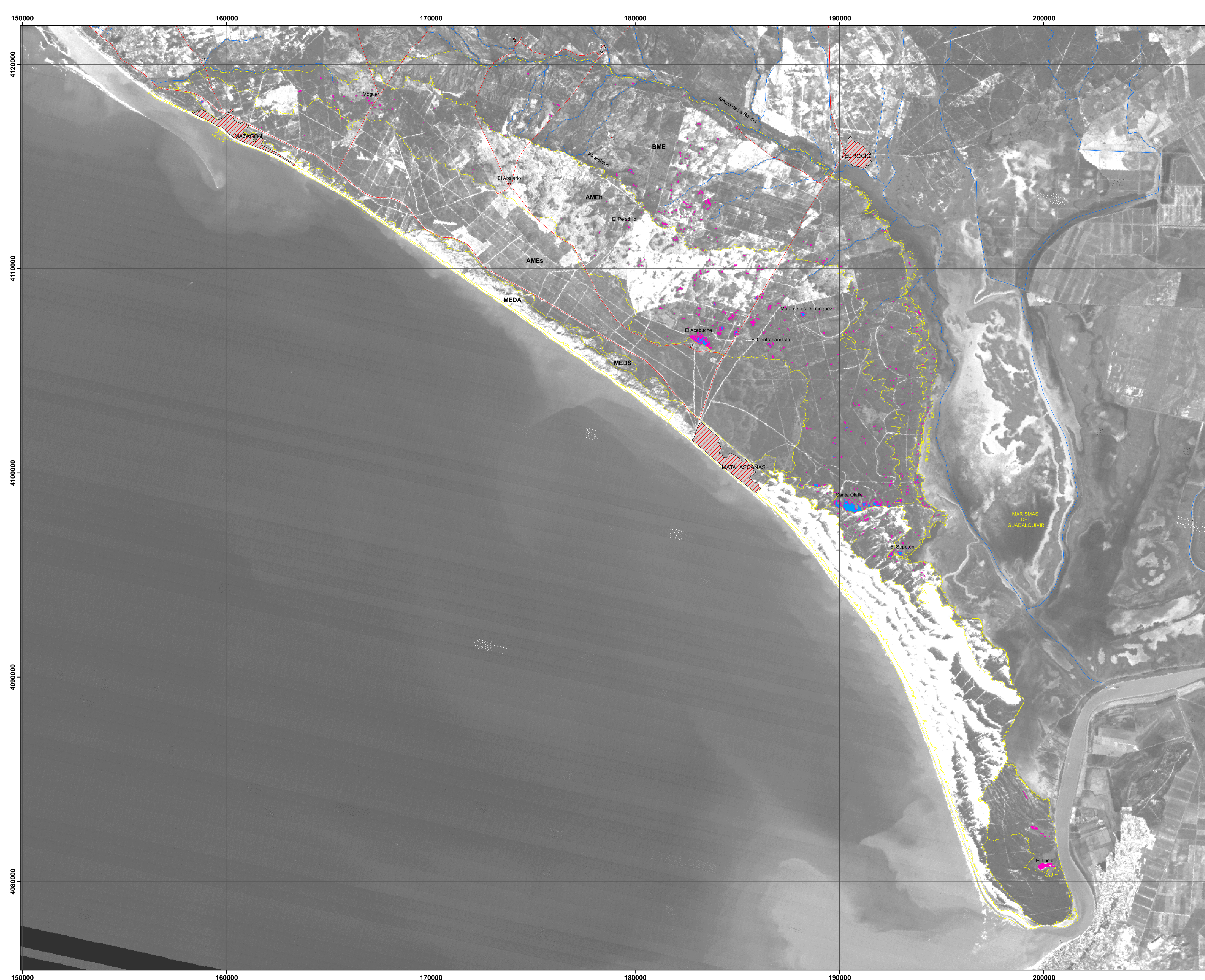
Cartografía de lámina de agua y superficies encharcadas. Febrero 1985. Landsat TM
